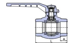
Кран сферичен
