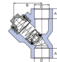
Възвратна клапа
