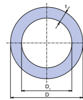
Труба Wavin Ekoplastik PP-R S 3,2 / PN 16 / SDR 7,4
