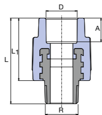
Преход с външна месингова резба
