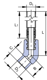
Връзка към радиатор – коляно 45°
