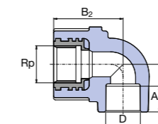
Коляно 90° с вътрешна месингова резба
