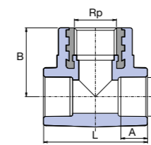
Тройник с вътрешна месингова резба
