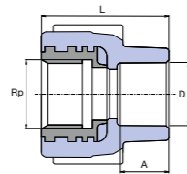
Преход за стена с вътрешна месингова резба
