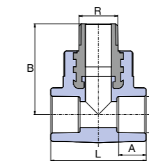
Тройник с външна месингова резба
