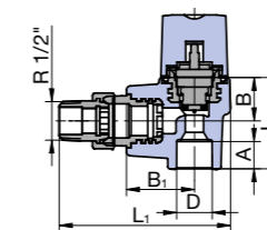
Термостатичен вентил за радиатор - ъглов
