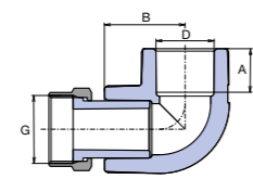
Коляно 90° с холендрова гайка
