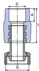
Преход с холендрова гайка и евроконус
