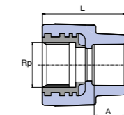
Преход с вътрешна месингова резба
