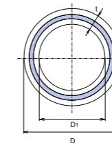
Труба Wavin Ekoplastik PP-RCT Fiber Basalt Clima 20 - 25 мм – S 4 / SDR 9 / PN 22 (изчислено)
