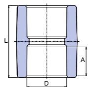
Муфа
