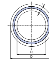
Труба Wavin Ekoplastik PP-RCT Fiber Basalt Plus 20 - 63 мм – S 3,2 / SDR 7,4 / PN 28 (изчислено)
