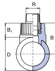
Седло - отклонение с външна резба
