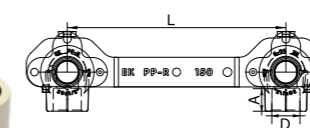
Колена за стена с фиксатор
