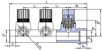
Колектор троен PP-RCT с регулиране
