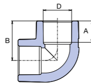
Коляно 90°
