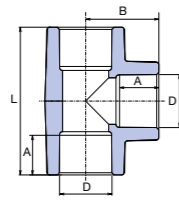
Тройник
