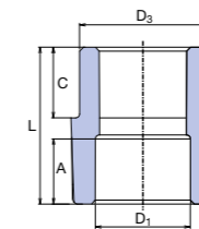
Редукция
