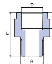
Преход с външна пластмасова резба
