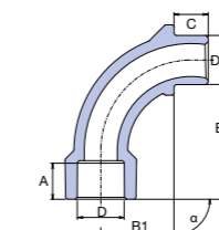
Дъга 90°
