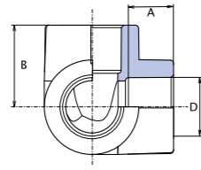
Трипътник
