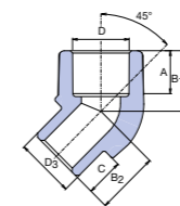
Коляно 45° мъжко / женско
