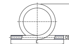
Компенсатор S 3,2 / SDR 7,4
