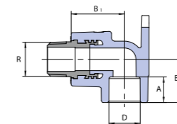
Коляно за стена с външна месингова резба
