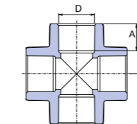
Четирипътник
