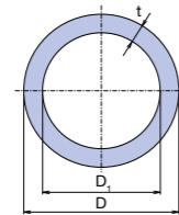
Труба Wavin Ekoplastik PP-R S 5 / PN 10 / SDR 11
