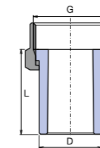
Холендър
