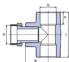
Тройник с холендрова гайка
