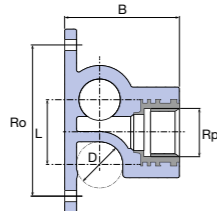
Ексцентрично коляно ляво
