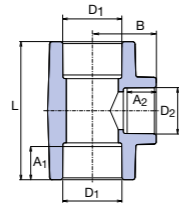
Тройник редуцирен
