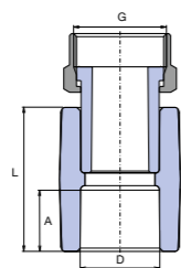
Муфа с холендрова гайка
