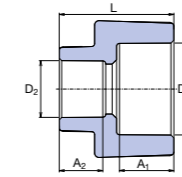
Редуктивна муфа
