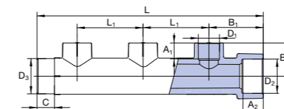
Колектор троен PP-RCT
