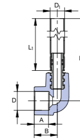
Връзка към радиатор – коляно 90°
