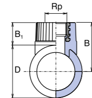
Седло – отклонение с вътрешна резба
