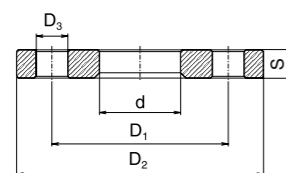
Фланец
